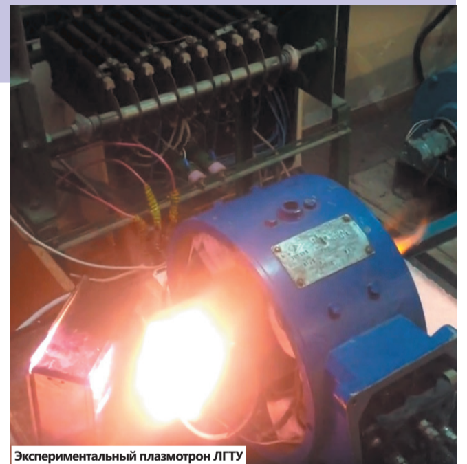
Экспериментальный плазмотрон ЛГТУ
